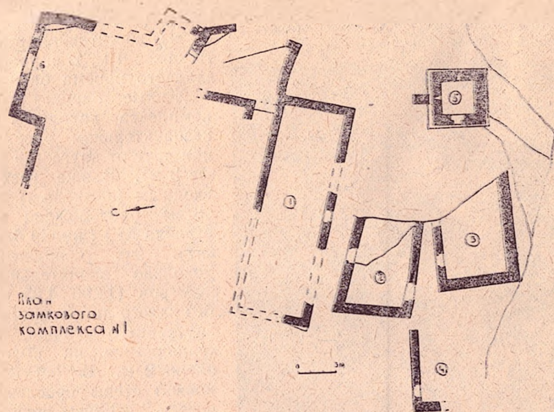
Рис. 5. План замкового комплекса № 1: 1 — жилая постройка (башня?) № 1; 2 — жилая башня № 2; 3 — жилая башня № 3; 4 — остатки жилой башни № 4; 5 — боевая башня; 6 — заградительная стена
