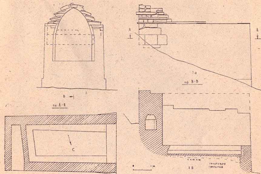
Рис. 10. План культовой постройки Эгичожского поселения
