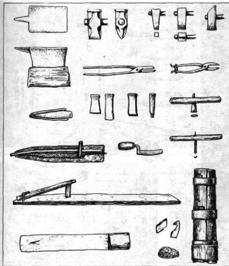
Рис. 169. Инструменты кинжальщика (по Е. М. Шилингу)
