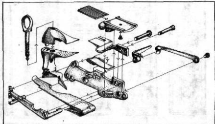
Рис. 204. Замок в разобранном виде
