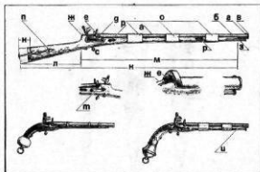
Рис. 5. Кремневое ружье и пистолет а — ствол; б — дульный срез; в — дульная часть; г — мушка; д — казенная часть; е — прицел; ж — хвостовик; з — шом- пол; и — шомпольное гнездо; к — ложа; л — приклад; м — цель; н — пятка или затыльник; о — обоймица; п — стрелка; р — гнездо или прорезь для ремня; с — спуск; т — замочная личина
