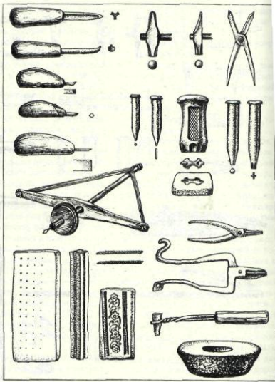
Рис. 171. Инструменты гравера (по Е. М. Шил- лингу).
