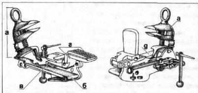
Рис. 6. Кремневый замок а — курок; б — подкурковая или боевая пружина; в — подогннная пружина; г — огниво и крышка полки; д — боковая планка
